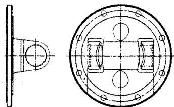
FLANGE YOE
