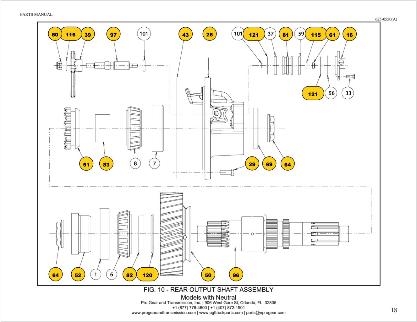
Fig. 10, ensamble de la flecha de salida trasera, modelos con neutral
